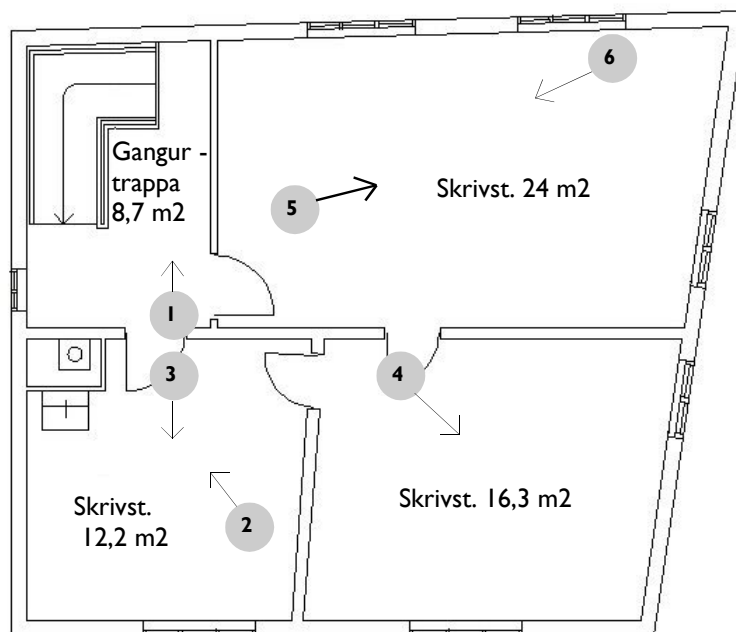
2. hædd / loft
