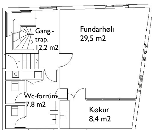
1. hædd
