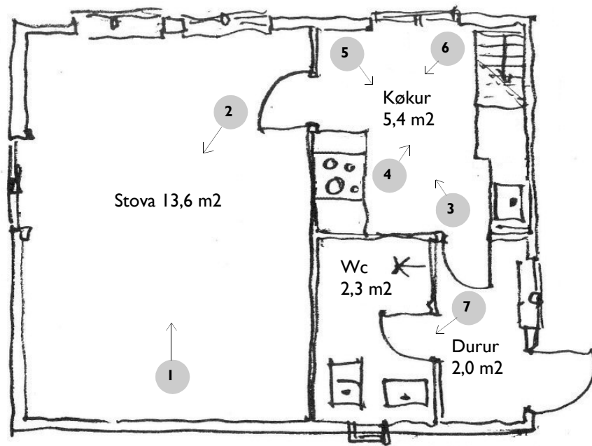
1. hædd
