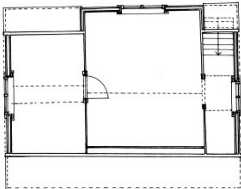
2. hædd / loft (1999)
