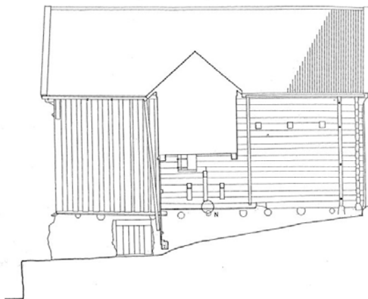
Norðursíða
